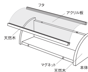
構造図
