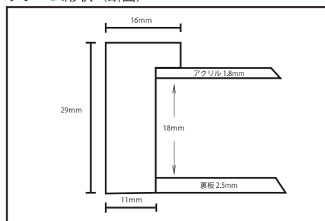
フレーム形状 (断面)
